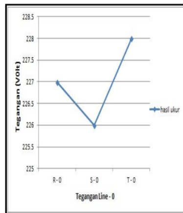
Gambar 3. Grafik pengukuran tegangan line to netral .
