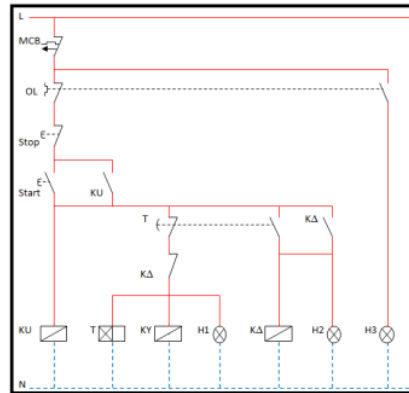
Gambar 2. Hasil perancangan rangkaian pengendali.
