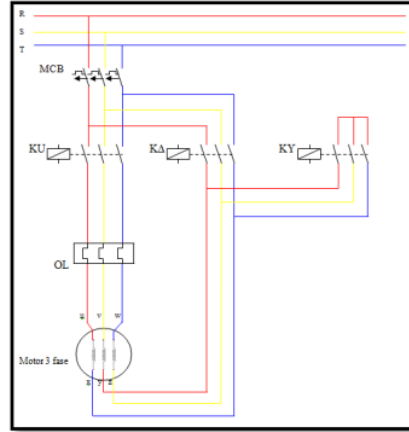
Gambar 1. Hasil perancangan rangkaian daya.
