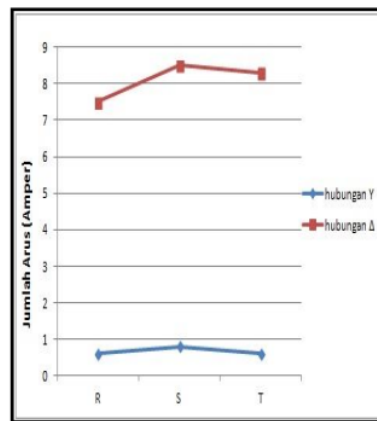
Gambar 4. Pengukuran fasa R, S, dan T dalam hubungan wye dan delta .
