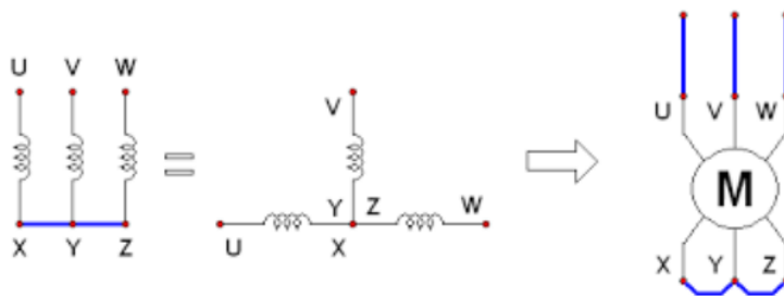
Gambar 1. Rangkaian delta motor induksi 3 fasa.
