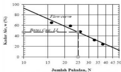
Gambar 1. Kurva pada penentuan batas cair tanah lempung
