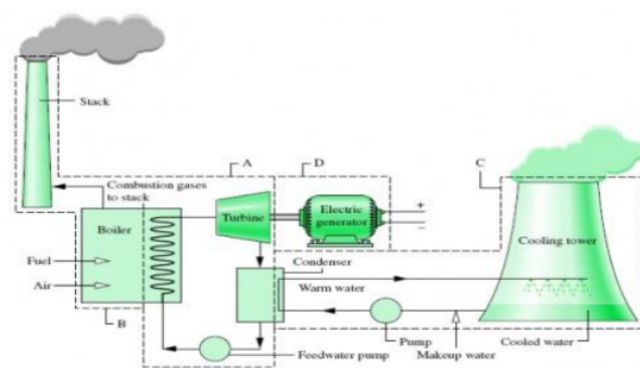
Gambar 1. Proses Konversi Energi PLTU
