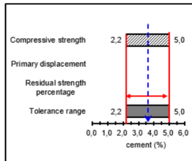
Gambar 8. Grafik kadar semen optimum
