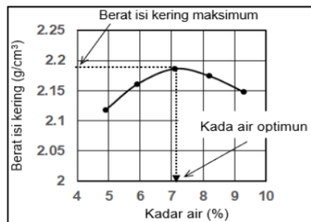
Gambar 1. Kurva hubungan antara kadar air dan kerapatan kering
