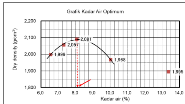
Gambar 6. Grafik Kadar air optimum
