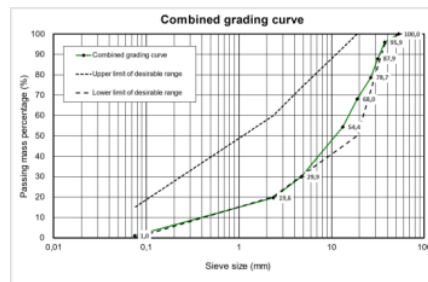
Gambar 3. Grafik gradasi agregat gabungan
