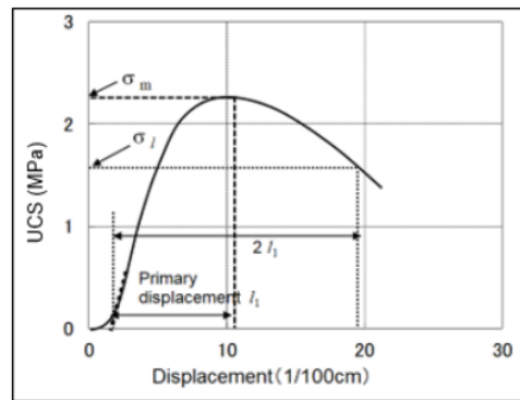
Gambar 2. Uji kuat tekan bebas
