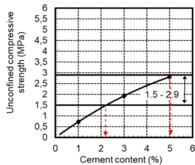
Gambar 7. Grafik hubungan KTB dan kadar semen
